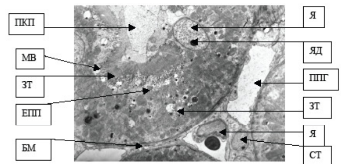
Рис. 3. Ультраструктура перитубулярних гемокапілярів та епітеліальних клітин канальців проксимального відділу нефрона білого щура зі стрептозототинним діабетом через один місяць лікування вітаміном С. 36. 6 000.
